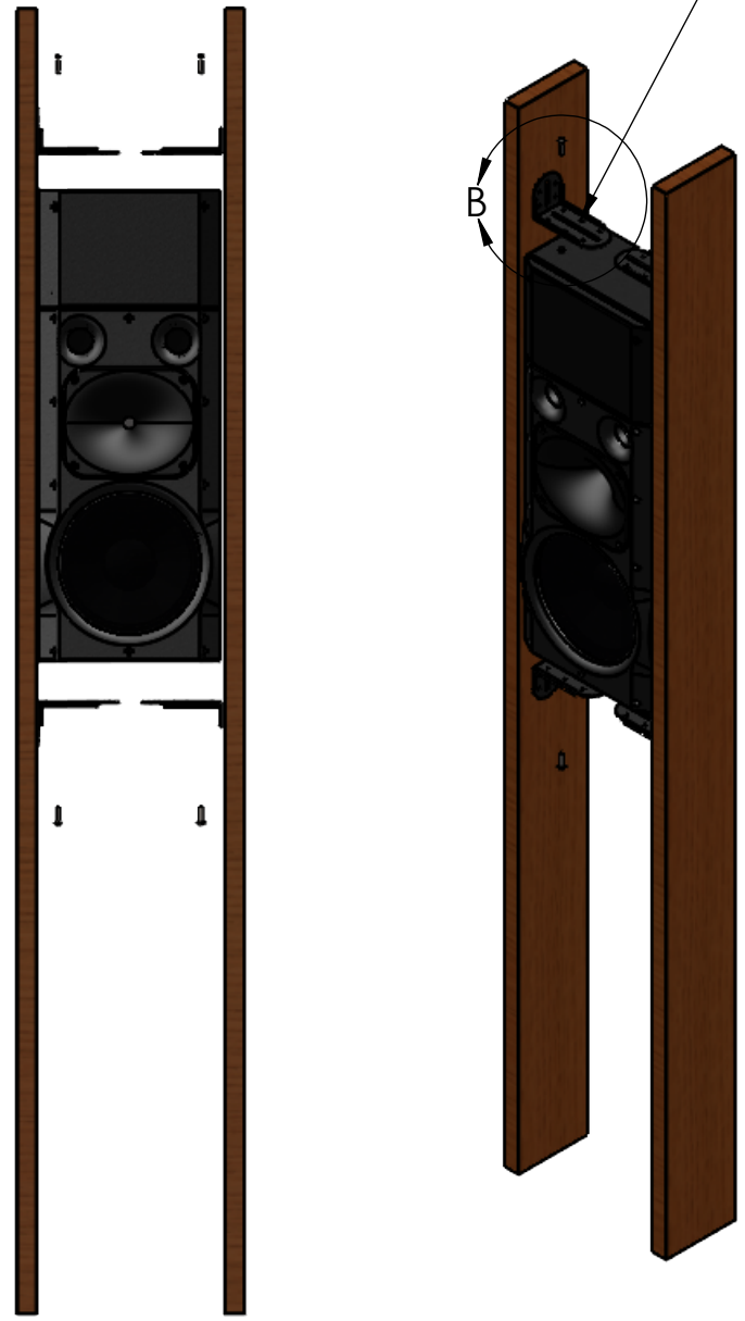
STUD MOUNT - STRAIGHT
