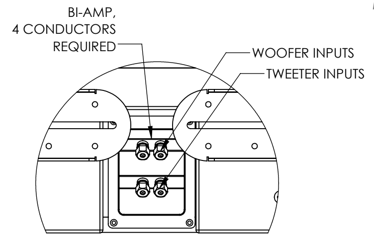
DETAIL A : INPUT TERMINALS SCALE 1 : 4
